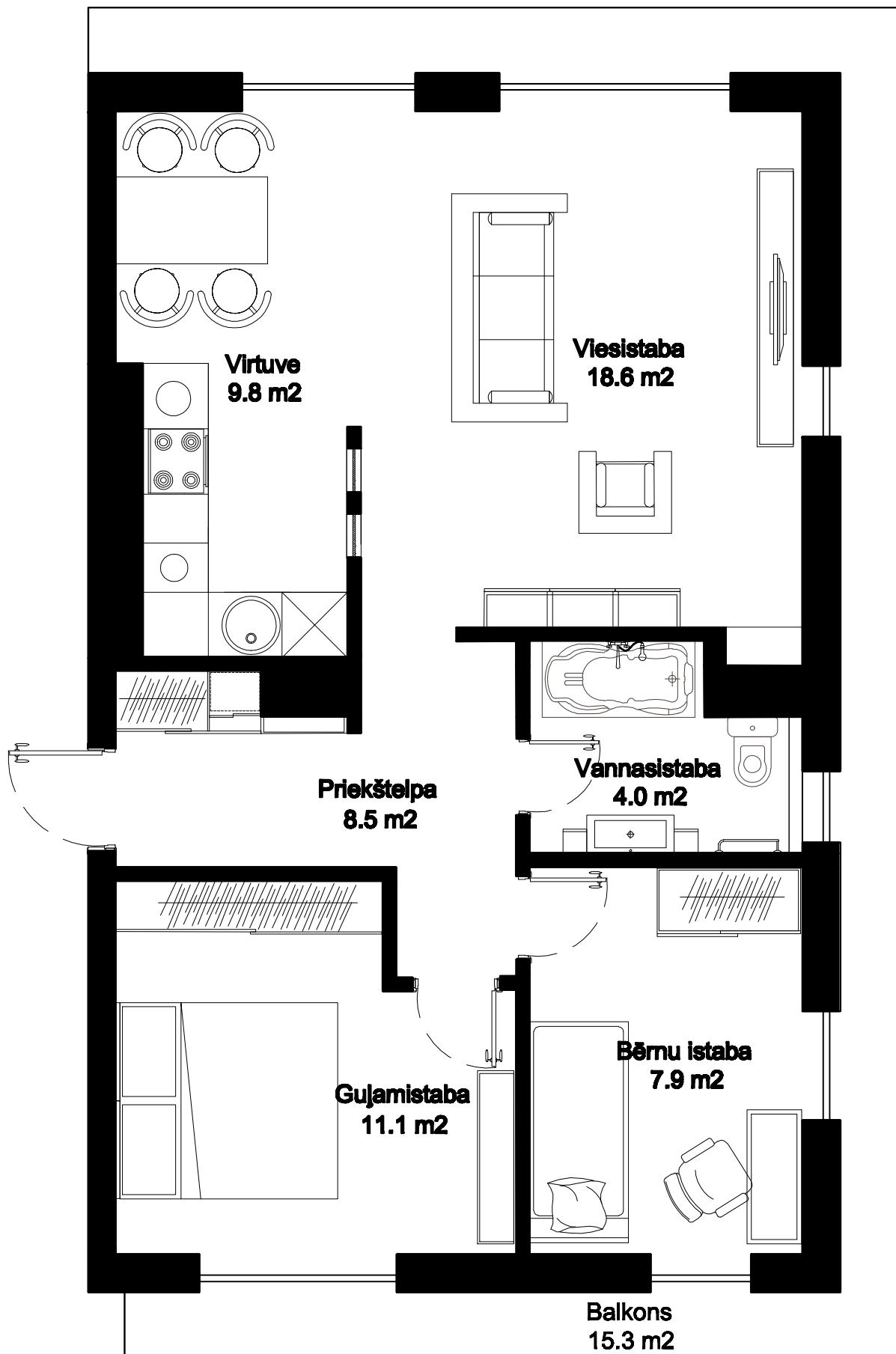
3.stāva plāns. 9.DZĪVKLIS
